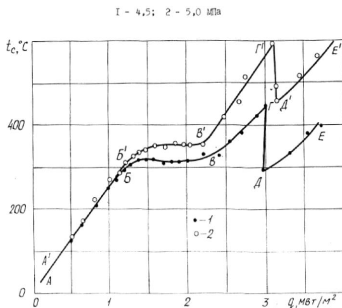
Рис.2. Зависимость t_c=f(q) для подъемного движения n -гептана при различных давлениях
